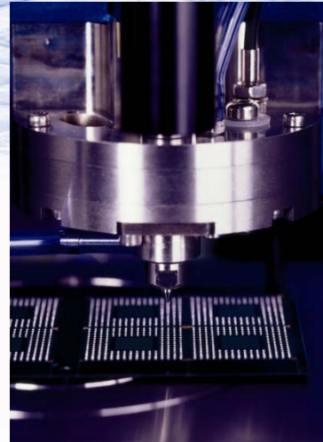
SB 2 -Jet Bond Head
